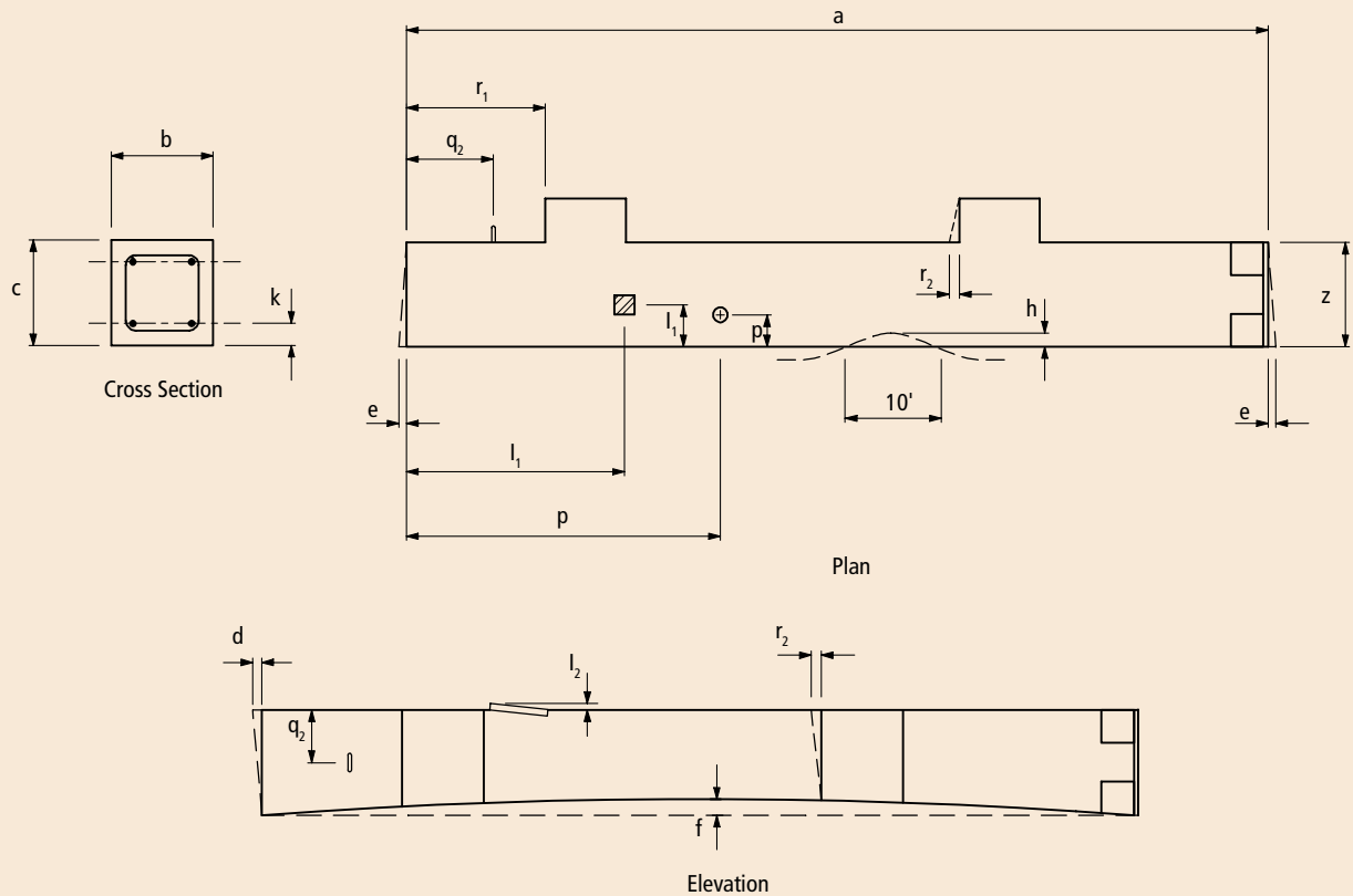
Fig. 4.6.6 Columns.
